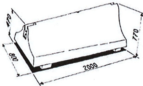
Endblock D Gewicht 950 kg
