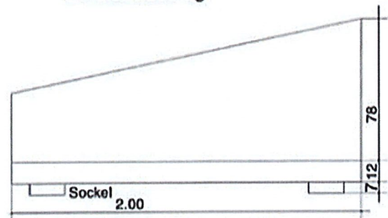
Übergangsblock F Gewicht 1200 kg
