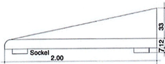
Endblock G Gewicht 700 kg
