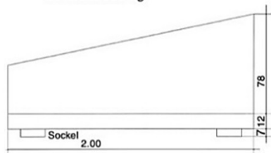
Übergangsblock F Gewicht 1200 kg
