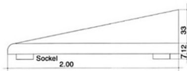
Endblock G Gewicht 700 kg
