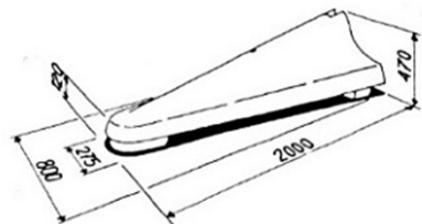
Endblock E Gewicht 500 kg
